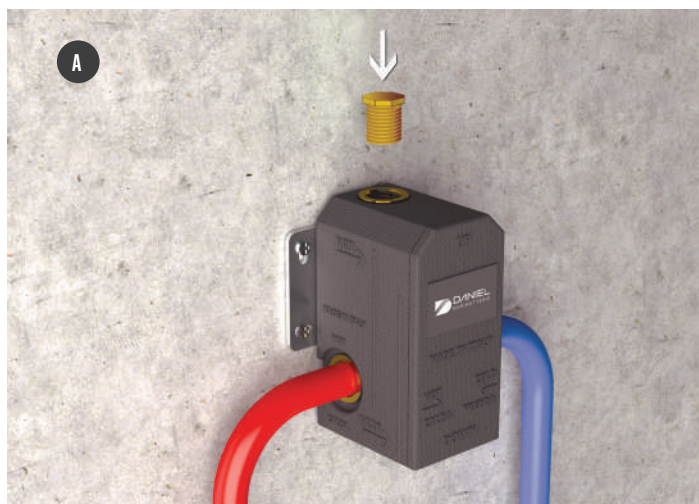
TAPPARE USCITA G 1/2 PLUG OUTLET G 1/2
