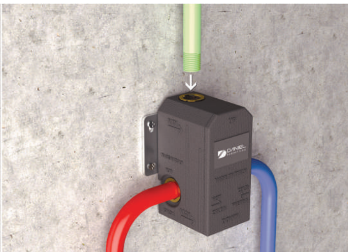
TAPPARE USCITA G 3/4 PLUG OUTLET G 3/4
